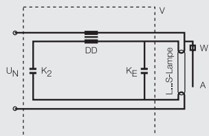
Рис. 5. Резонансная схема зажигания
