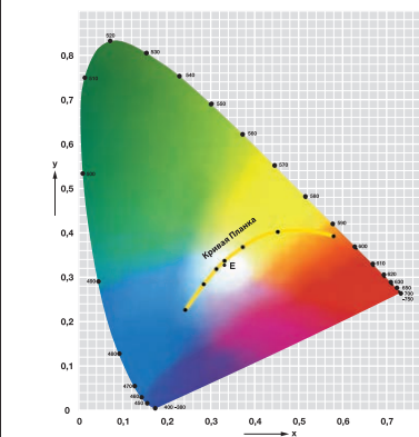
Цветовой график (локус) по стандарту DIN 5033
