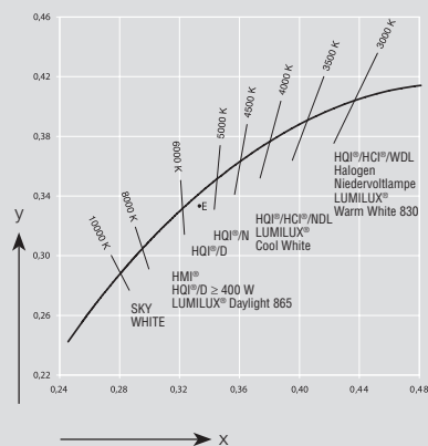
Фрагмент цветового графика с кривой Планка
